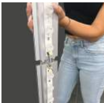
3) Inserire il secondo profilo laterale nell'inserto di quello sottostante
